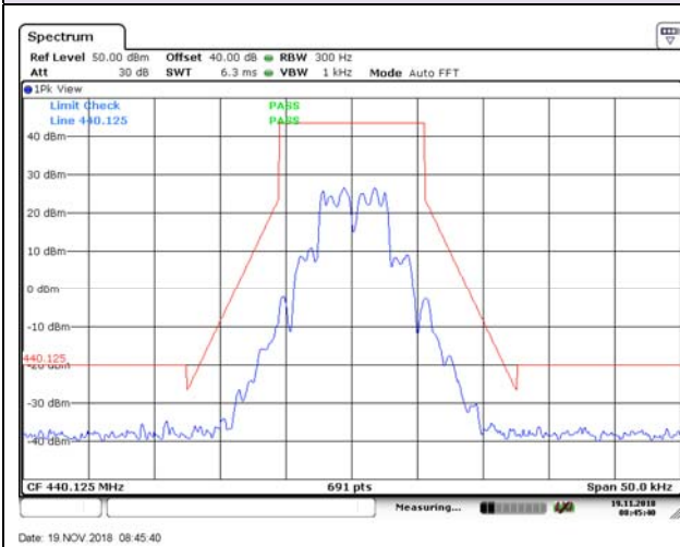
440.125MHz GMSK
