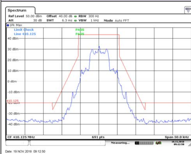
410.125MHz GMSK
