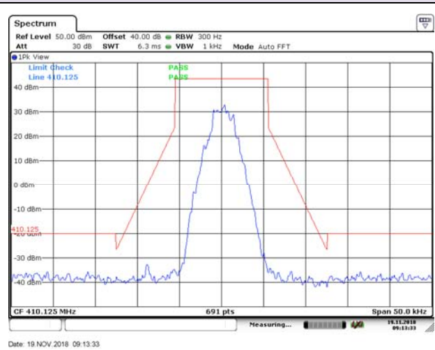
410.125MHz 4FSK
