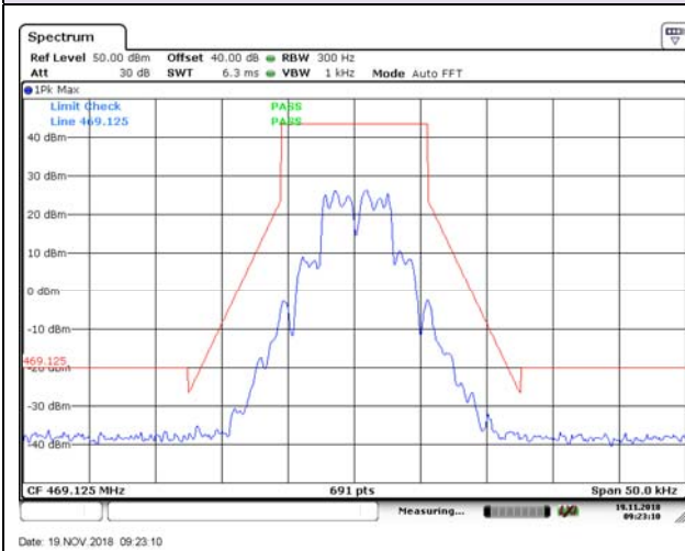
469.125MHz GMSK
