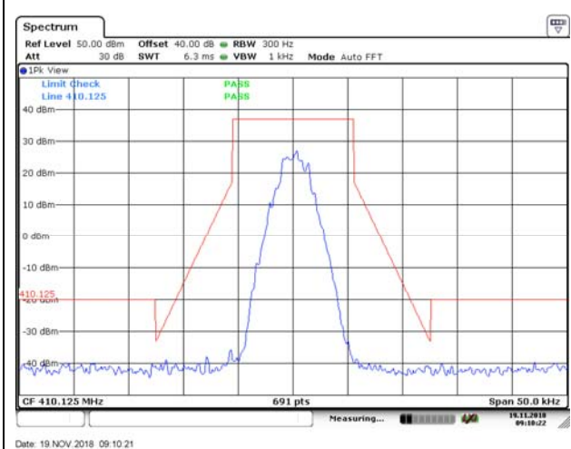
410.125MHz 4FSK
