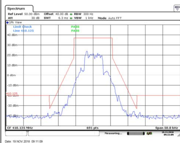
410.125MHz GMSK
